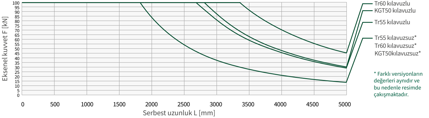
Kritik burkulma kuvveti ZA-100
