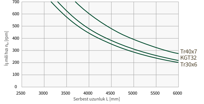
Kritik Bükme hızı ZA-25
