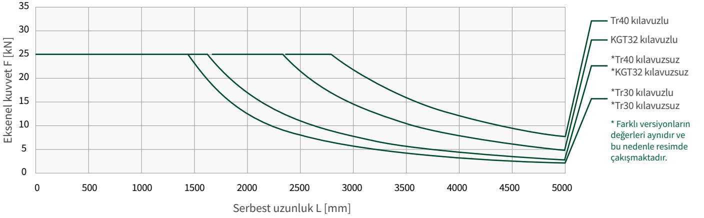
Kritik burkulma kuvveti ZA-25
