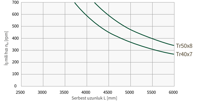
Kritik Bükme hızı ZA-50
