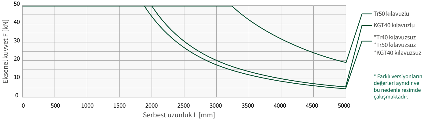
Kritik burkulma kuvveti ZA-50
