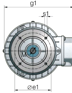
B14: İç dişli flanş C: Küçük flanş
