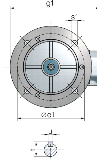
B5: Geçiş delikli flanş
