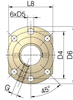
Delik modeli 1 DIN 69051'e göre
