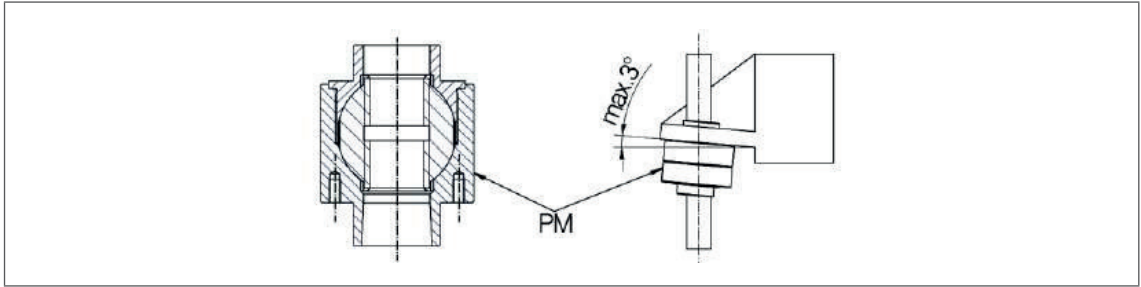
Şek. 10: İstisna: Sarkaç somununun (PM) maksimum eğim açısı 3°'dir, diğer tüm somunları dik açıyla monte edin.
