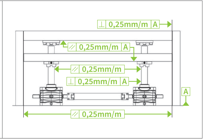
Şekil 8: Montaj hassasiyeti: paralellik ve diklik
