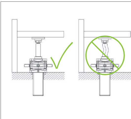
Abb. 7: Seitliche Belastung der Spindel unzulässig.
