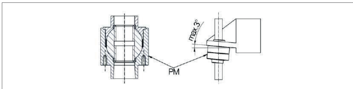
Abb. 10: Ausnahme: Maximaler Neigungswinkel der Pendelmutter (PM) ist 3°, alle anderen Muttern rechtwinklig montieren.
