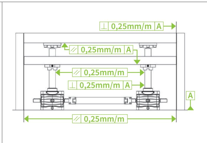
Abb. 8: Einbaugenauigkeit: Parallelität und Rechtwinkligkeit
