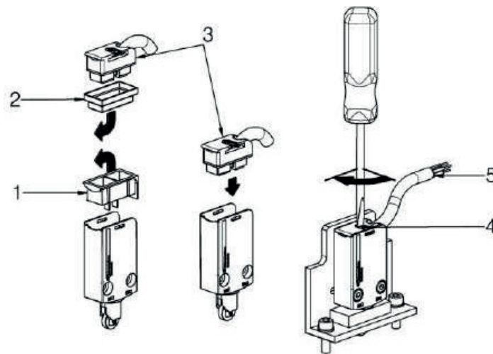
Abb. 14: Anschlussstecker am Endschalter montieren
