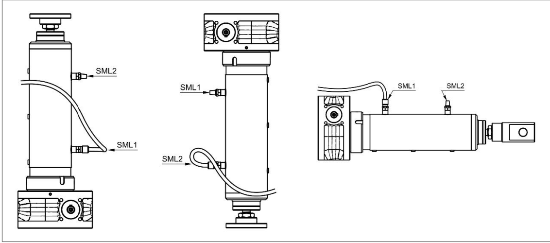
Şek. 17: Otomatik yağlama ile havalandırma konumu
