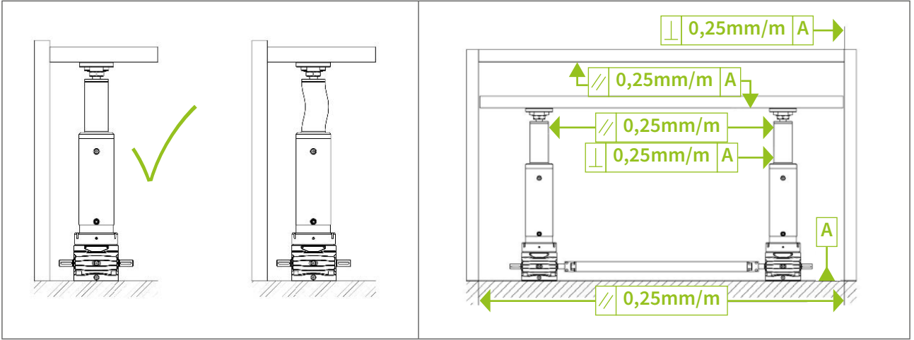
Şek. 5: Montaj başlığı üzerindeki maksimum yanal yüke dikkat edin
