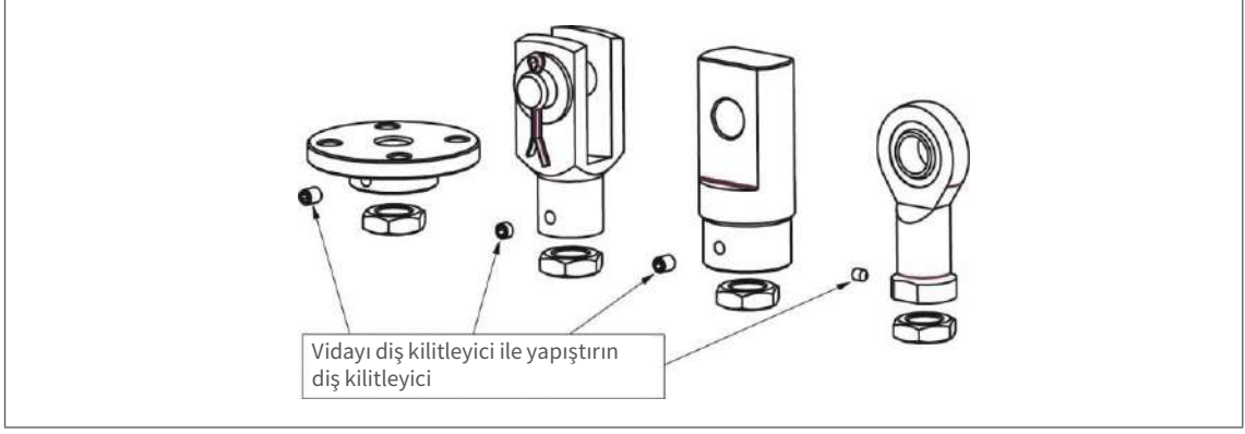
Şek. 7: Pozisyonu ayarladıktan sonra flanşları, , döner yatağı ve bilyeli mafsalları sabitleyin.
