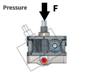
Permissible nominal load 25 kN
